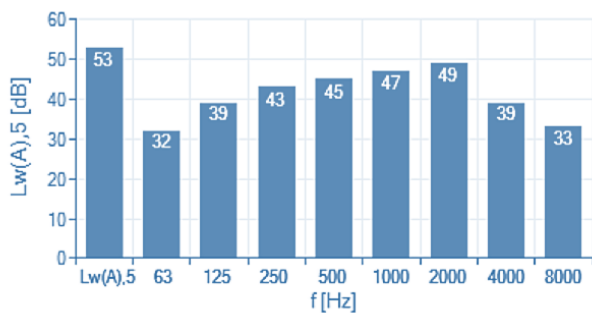
Akoustisch, aanzuigzijde L w (A) (bij 200 m 3 /h)
