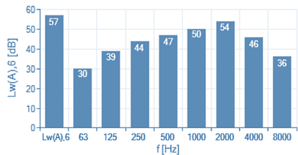
Akoustisch, uitblaaszijde L w (A) (bij 200 m 3 /h)
