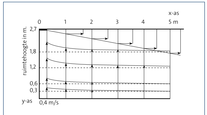
Fig. 3.5 Snelheidsopbouw retourwervel in de y-richting vlak patroon
