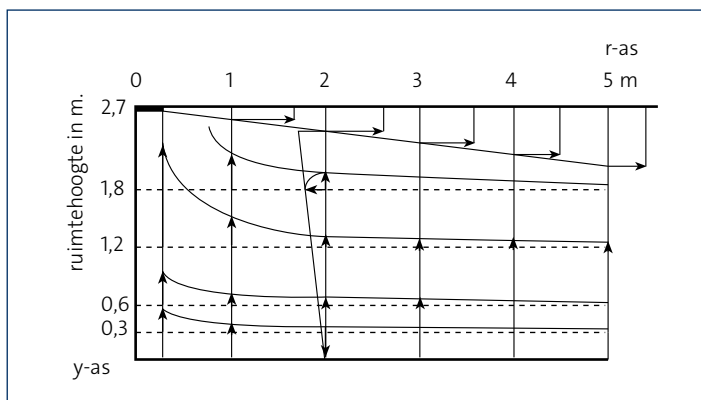
Fig. 3.2 Snelheidsopbouw retourwervel in de y-richting radiaal
