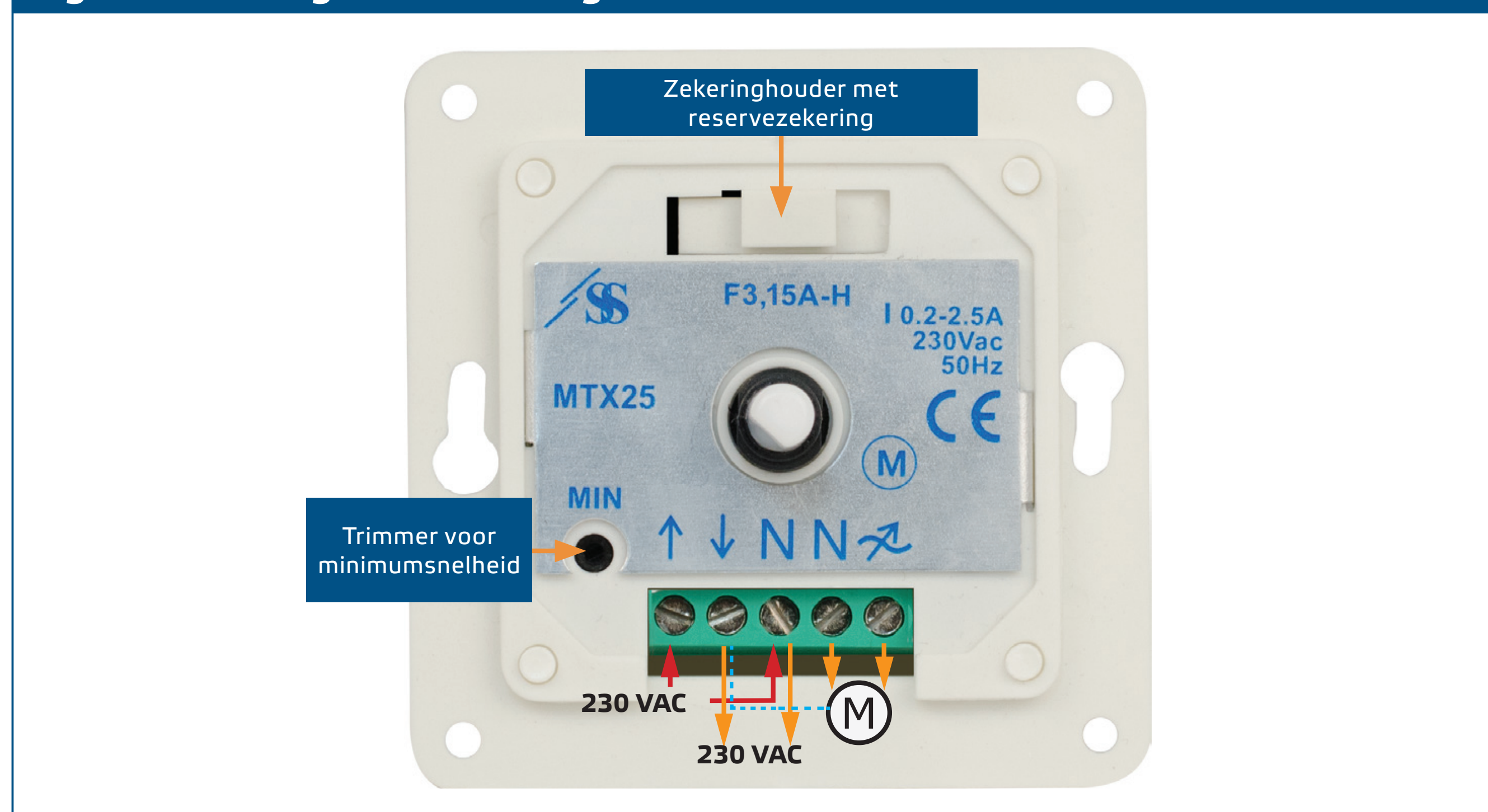
Fig. 1 Bedrading en aansluiting
