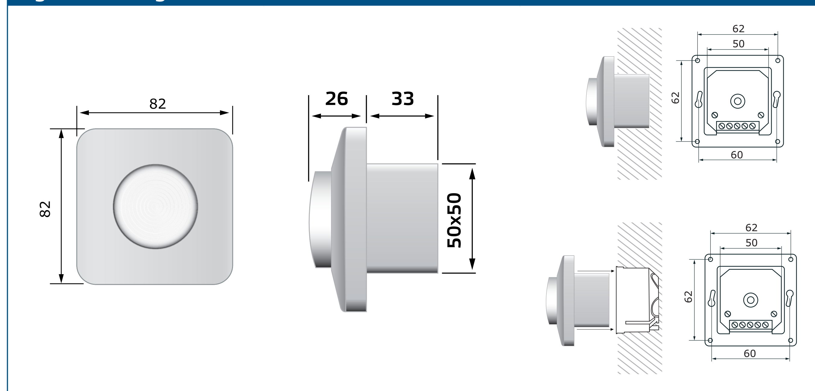
Fig. 2 Afmetingen - inbouw
