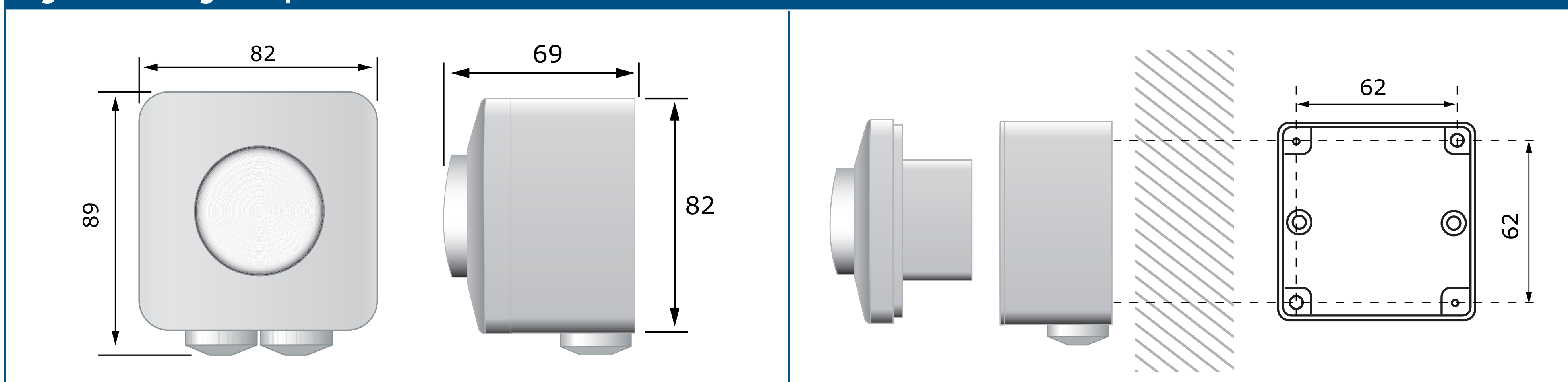
Fig. 3 Afmetingen - opbouw
