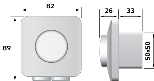
Fig. 2 Montageafmetingen - inset montage
