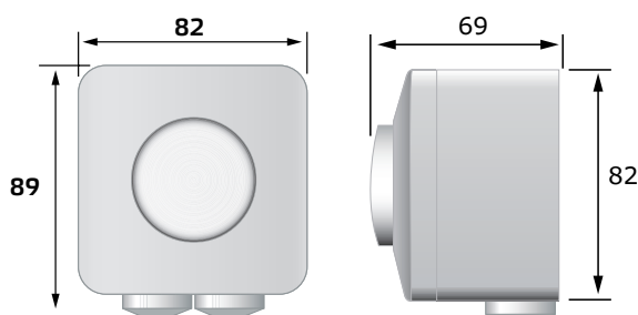
Fig. 3 Montageafmetingen - opbouw montage
