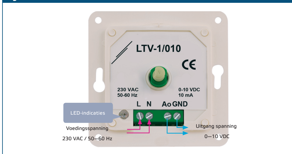
Fig.1 Aansluitschema
